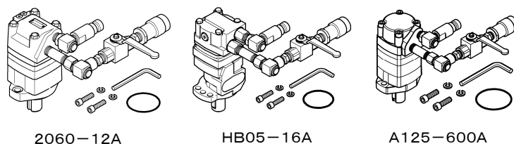
油圧モータ組
