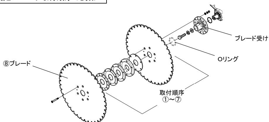
切断幅とスペーサ取付順序の関係
