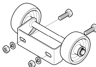
ベース用キャスター BK - 591C
