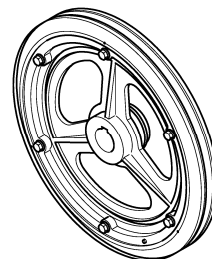
ブーストドライブプーリ
