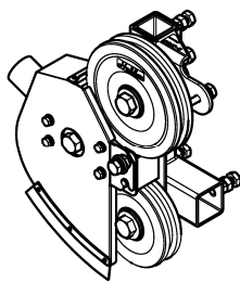
インテークガイドプーリ組S
