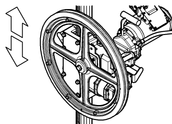
送りスイッチ 「切削」 引張力ボリューム 「5～6」
