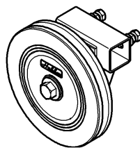
φ200、φ220、φ250 樹脂ガイドプリーGX組
